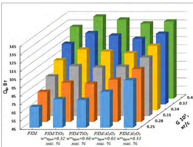
Значення холодопродуктивності для робочих тіл (РХМ/наночастинки) за різних витрат
