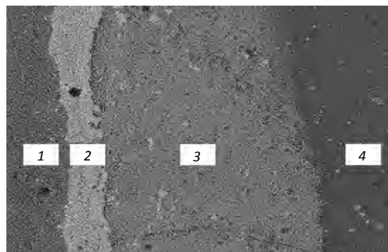
Поперечний переріз покриття \text{Ti-NbN-Al}_2\text{O}_3 на поверхні різального елемента: 1 – основа; 2 – \text{Ti} ; 3 – \text{NbN} ; 4 – \text{Al}_2\text{O}_3
