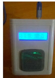
Зовнішній вигляд частотного вимірювача концентрації пилу
