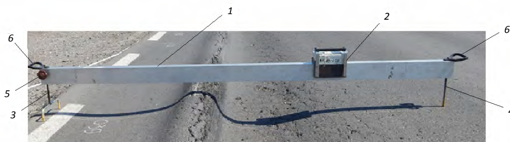
1 – балка; 2 – рухома каретка; 3 – ліва опора; 4 – права опора; 5 – фіксатор лівої опори; 6 – ручки для переноски колієвимірювача
