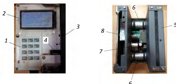
1 – клавіатура; 2 – дисплей; 3 – відкидна ручка для переноски; 4 – флеш-пам'ять; 5 – корпус; 6 – ролики приводу; 7 – електродвигун; 8 – лазерний датчик
