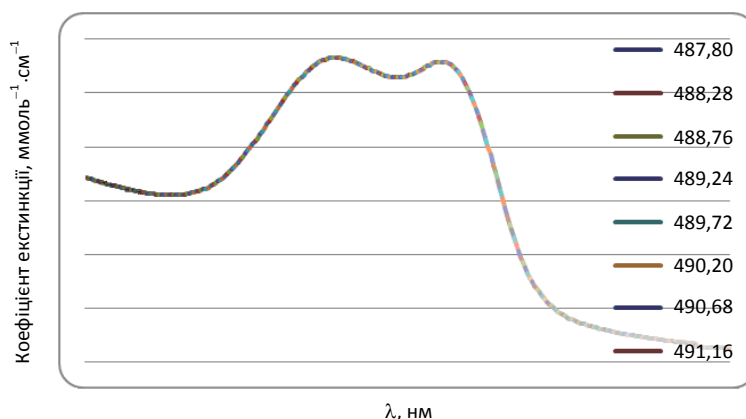
Спектр поглинання нітрозилгемоглобіну крові здорових донорів, побудований за даними мілімолярних коефіцієнтів екстинкції
